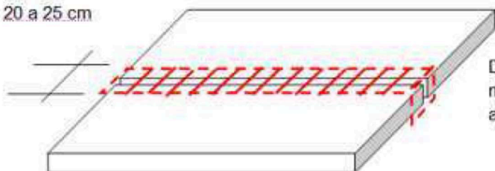
Figura 1. Esquema aplicação manta geotêxtil (Fonte: Transmar consultoria e engenharia)
