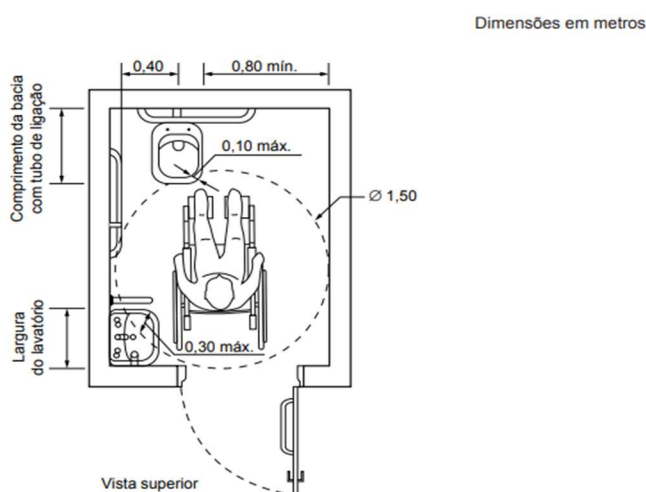
Figura 99 – Medidas mínimas de um sanitário acessível
