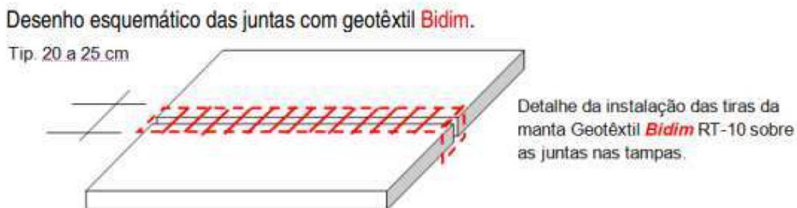
Figura 1. Esquema aplicação manta geotêxtil (Fonte: Transmar consultoria e engenharia)
