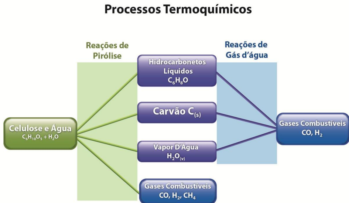
Figura 18: Sistema Innova – Esquema dos processos termoquímicos
