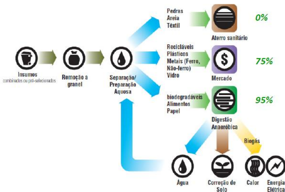
Figura 19: Sistema ArrowBio – Esquema do processo
