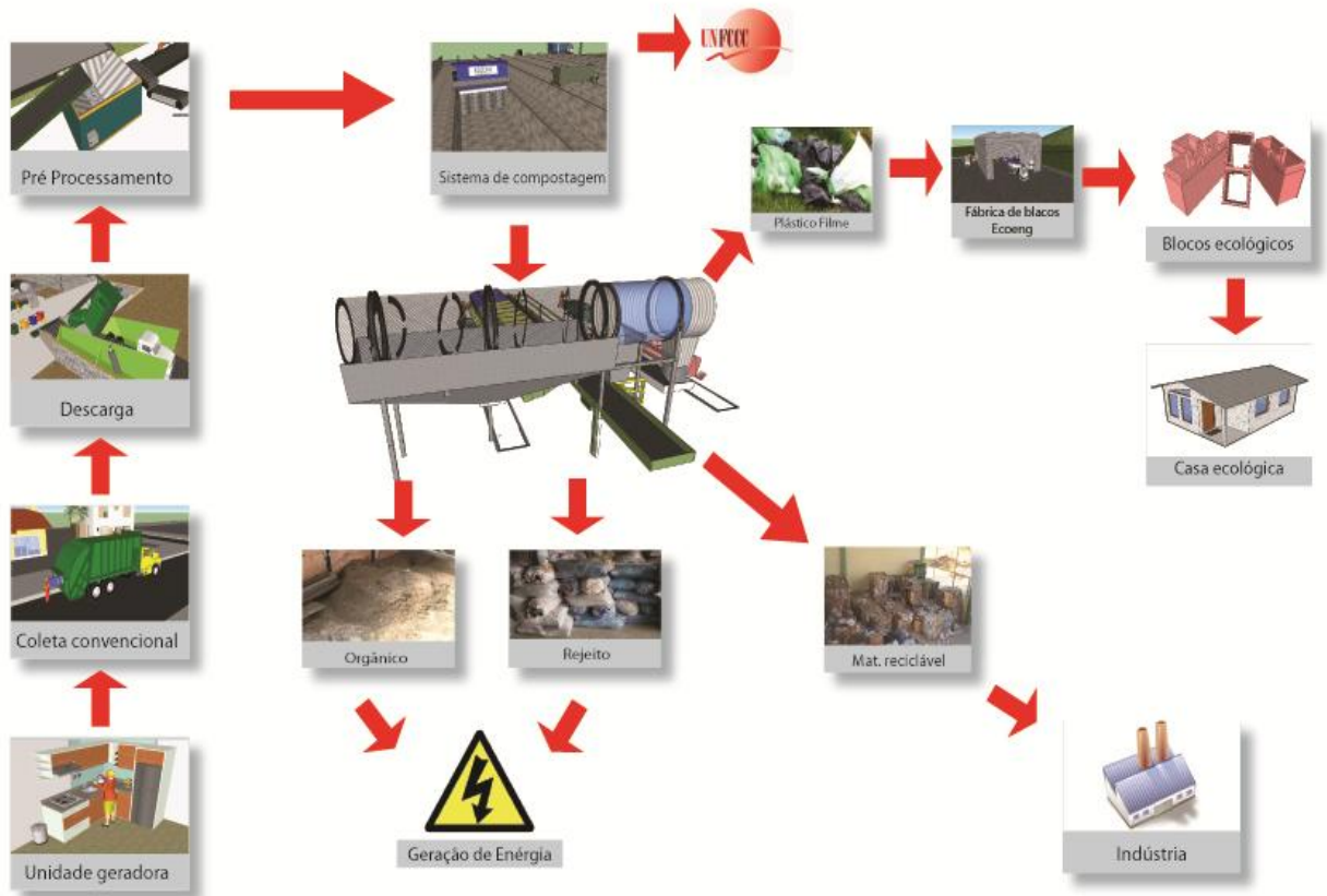
Figura 12: Sistema Eco Eng - Tratamento e destinação Final de Resíduos Sólidos
