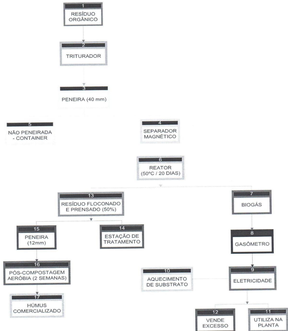
Figura 22: Fluxograma do processo contemplado na tecnologia Dranco
