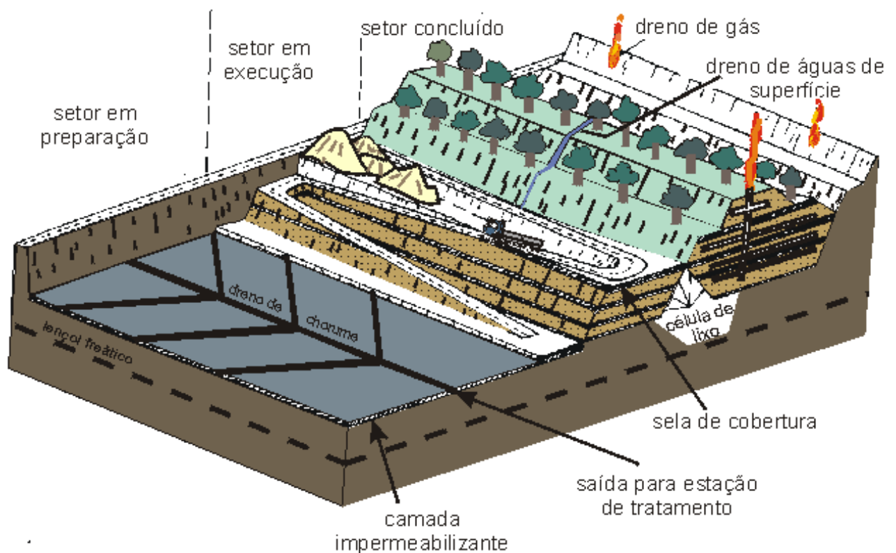
Figura 3: Estrutura padrão de aterros sanitários
